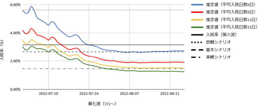
第七波の入院率（東京都）
