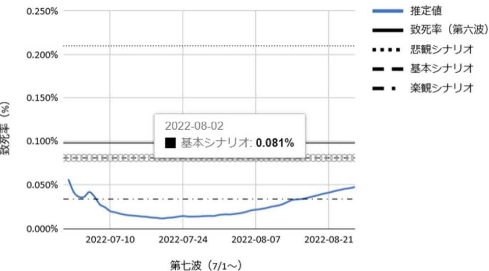
第七波の致死率（東京都）
